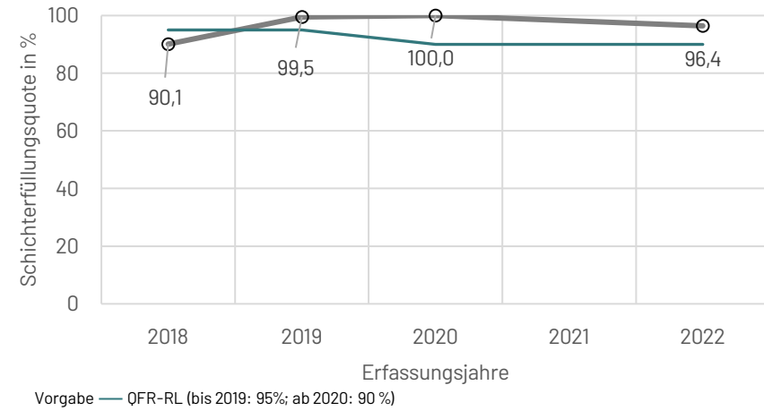
Entwicklung Schichterfüllungsquote Klinikverbund Allgäu, Klinikum Kempten (771222) und Vorgabe QFR-RL (2018-2022)
